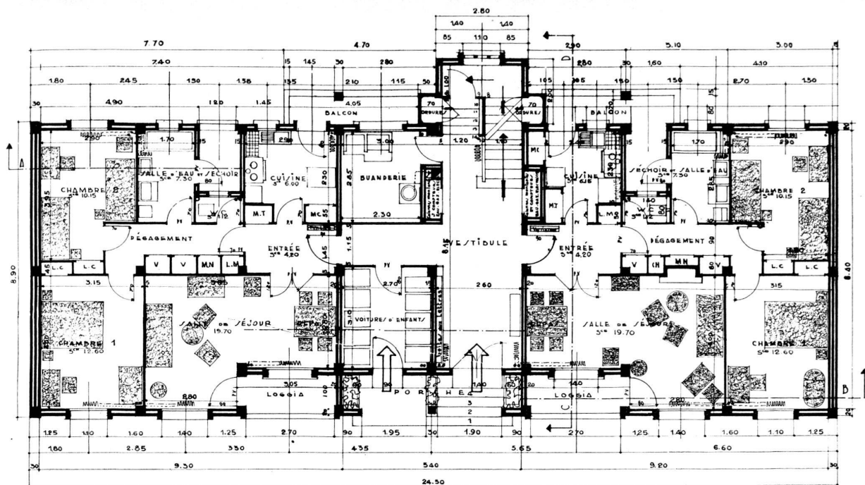
Plan à rez-de-chaussée. Molinié, Sarce, Chevenot, architectes.
