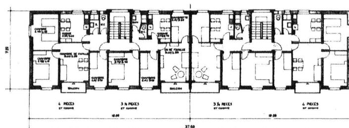
PLAN D'ETAGE
