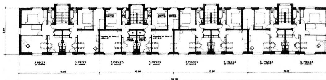
PLAN D'ETAGE
