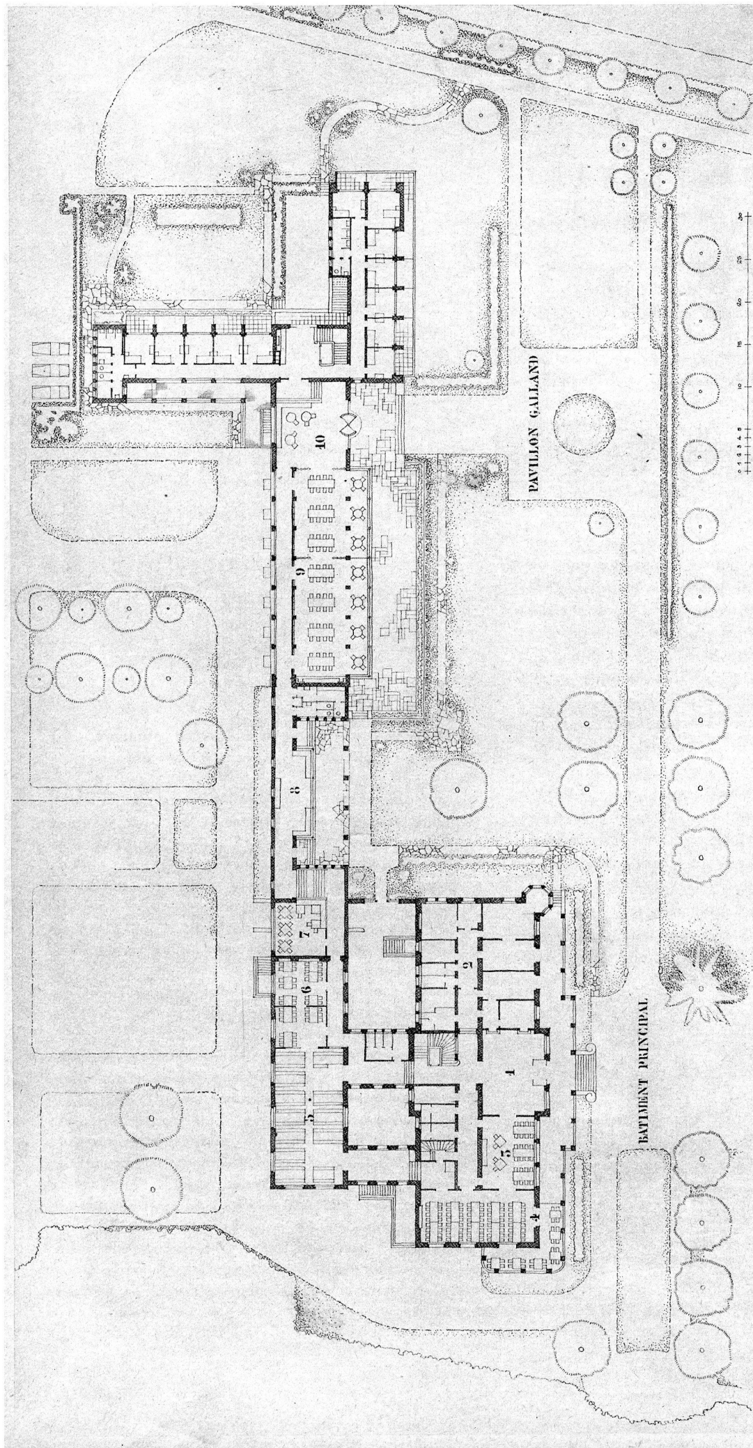
PLAN GÉNÉRAL DU REZ-DE-CHAUSSEE
