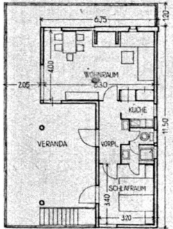
Obergeschoß.
