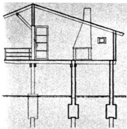
Plans et coupes de la construction.
