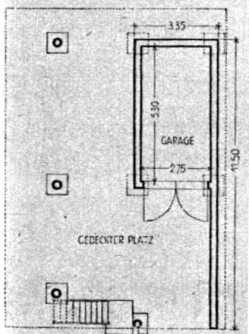
Maisonnette de vacances au bord du lac de Sempach.
