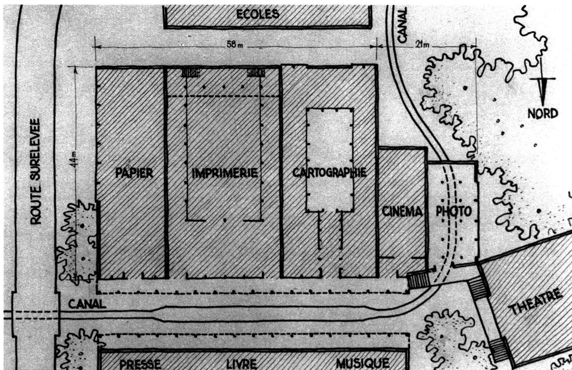
Plan général.
