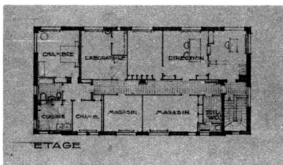
Plans du rez-de-chaussée et de l'étage.
