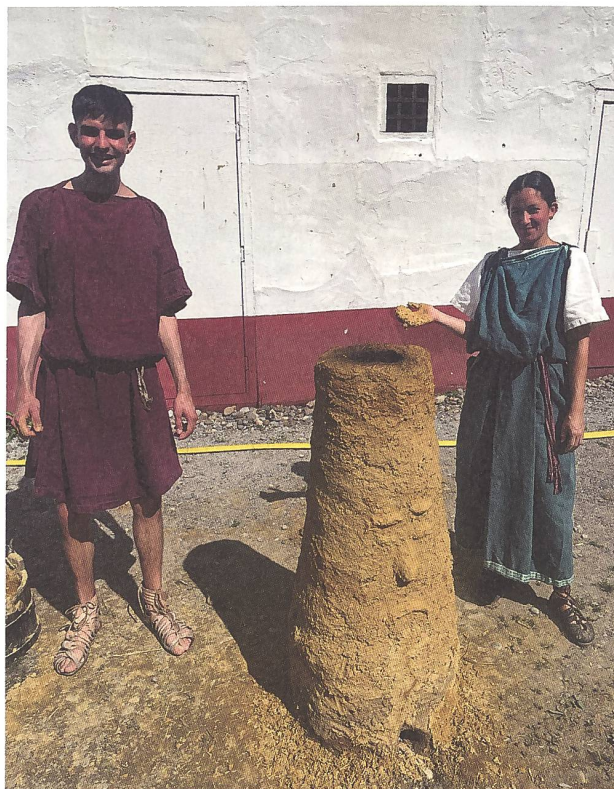
Abb. 7: Die Geschichtsvermittlerin Isabella Cadilek und der Geschichtsvermittler Pirmin Bischoff beim Aufbau des Rennofens am Handwerks-Parcours.
