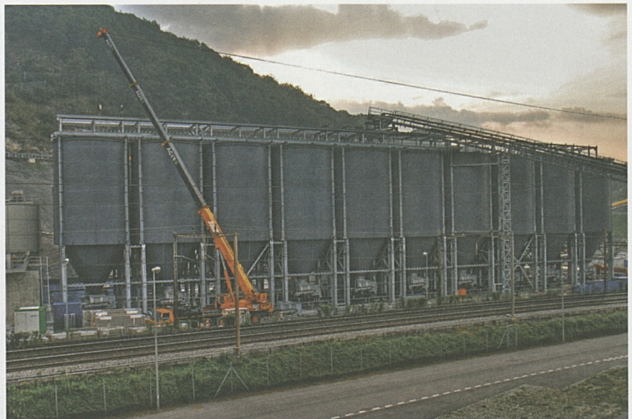
La batteria di sili dell'impianto per la gestione del materiale estratto.
