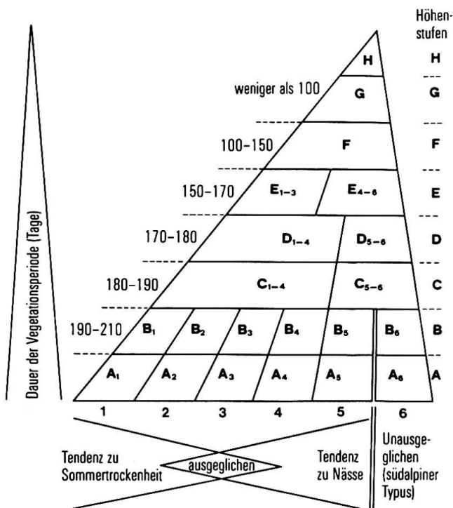
Niederschlagshaushalt
