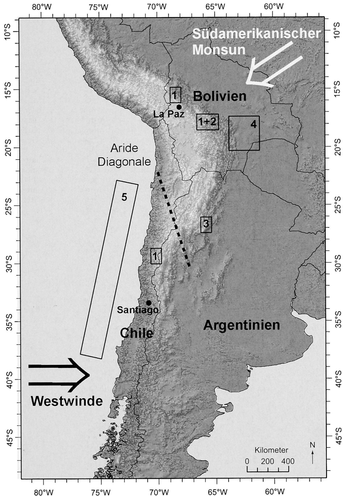
Abb. 1: Lage der in diesem Heft vorgestellten Untersuchungsgebiete (1 = ZECH et al., 2 = IMHOF et al., 3 = SCHELLENBERGER, 4 = MAY, 5 = STUUT et al.)
