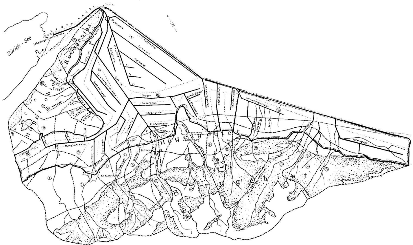
Abb. 5 Plan der modernen Gewässerkorrektur der linksseitigen Linthebene. Aus dem Schlußbericht der Melioration der Linthebene, 1966.
