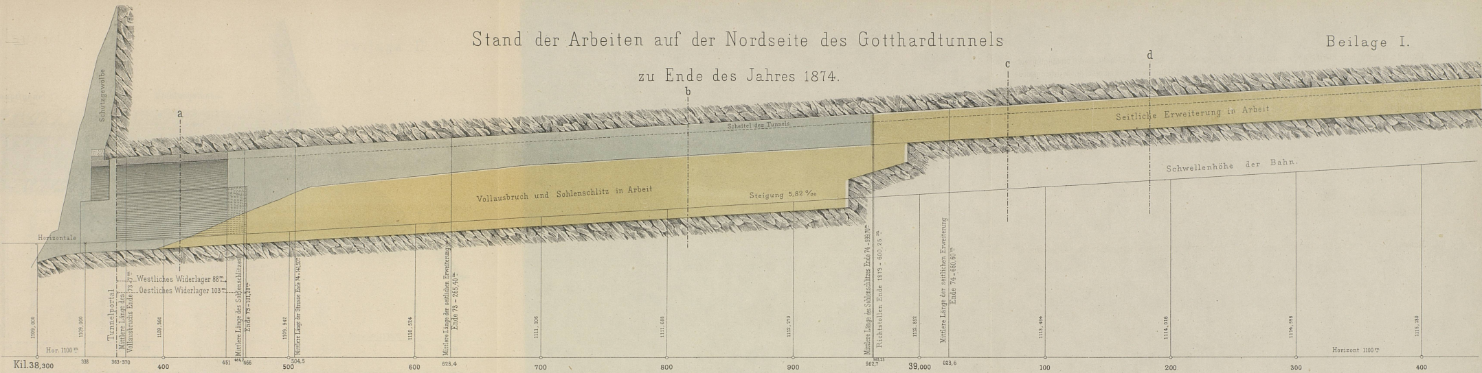
Fortsetzung des Längenprofils.
