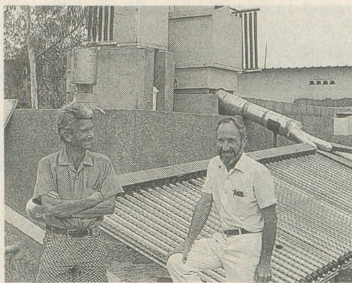
Jean-Paul Murset et le Dr Ken Elliott devant le stérilisateur solaire fonctionnant à l'hôpital, créé par le Dr Elliott à Djibouti. Jean-Paul vient de repartir pour la 7e année consécutive, afin d'assurer la bonne marche des instruments de l'hôpital. Photo Willy Randin
