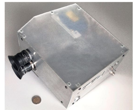
Fig. 1: Système d'acquisition pushbroom utilisant le capteur Headwall.
