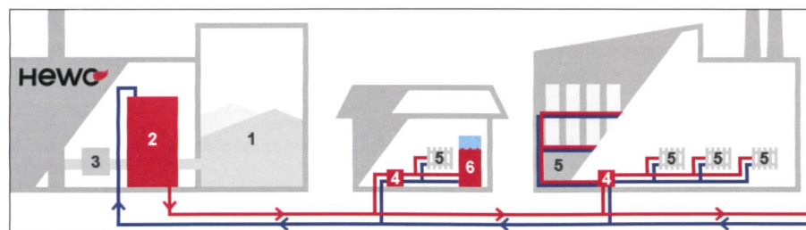
Abb. 1: Wärmekreislauf 2 .
