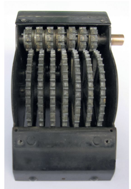
Abb. 4: Ein Blick ins Innere des Volksrechners zeigt die Zahnräder des Einstellwerks (unten) und des Ergebniswerks (oben).
