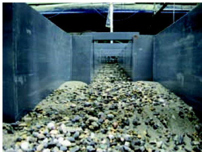
Fig. 2: Laboratoire LCH: Essai sur modèle physique en laboratoire simulant les conditions en l'absence du seuil: vue du chenal principal sur l'embouchure élargie de son affluent; suite à l'élargissement de l'embouchure, la morphologie du fond se diversifie, créant des conditions favorables à l'émergence de nouveaux habitats et à la libre circulation des poissons (LCH/EPFL).
