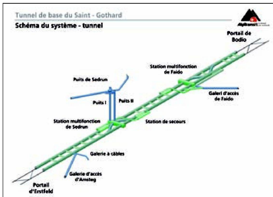
Fig. 1: Le système de tunnel au Gothard.
