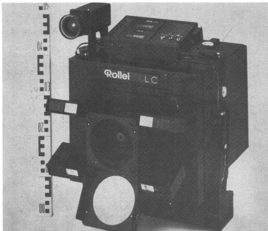
Rolleif LFC: Aufnahmekamera für ein Industriemesssystem hoher Präzision
