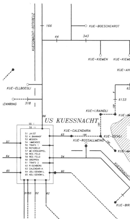
Abb. 2: Ausschnitt aus dem Mittelspannungsschema der Centralschweizerischen Kraftwerke AG (CKW).
