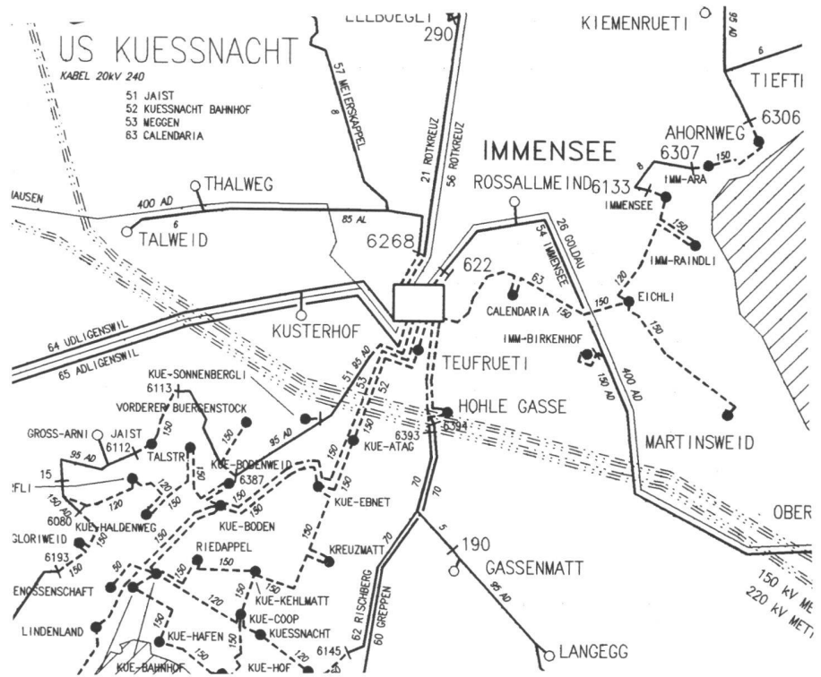
Abb. 3: Ausschnitt aus dem Verteilnetz-Planwerk der Centralschweizerischen Kraftwerke AG (CKW).
