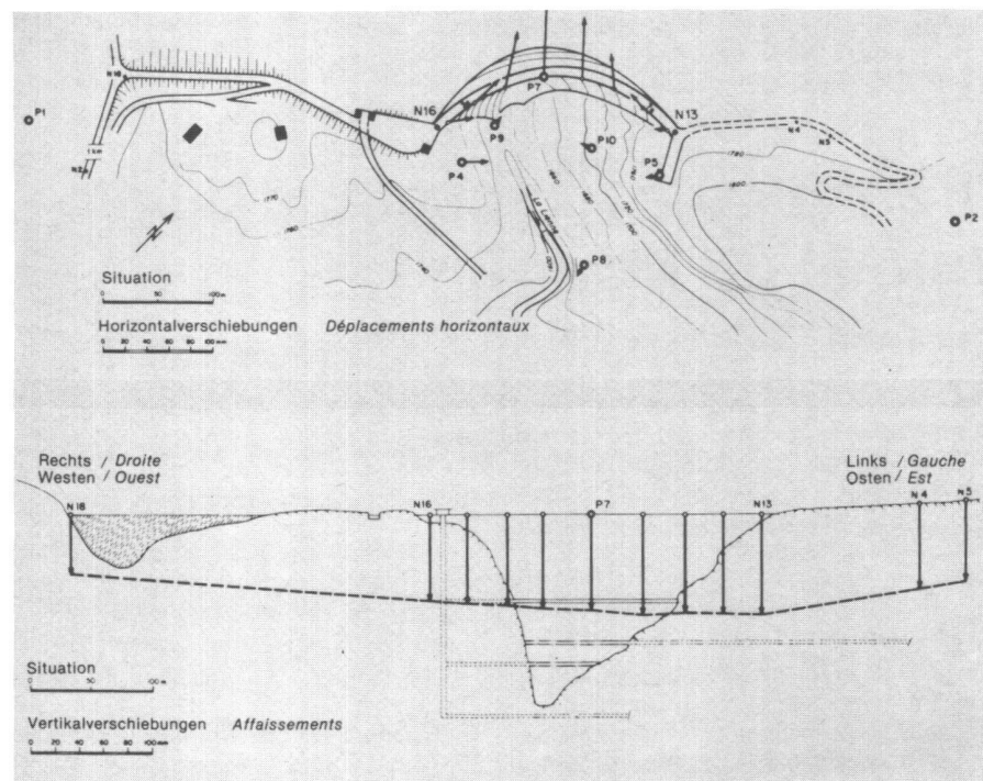
Abb. 5: Die Staumauer von Zeuzier (1777 m.ü.M.) wurde zwischen 1954 und 1957 errichtet. Ihre Höhe beträgt 156 m. Vom Zeitpunkt der Fertigstellung bis zum Jahre 1976 verhielt sich die Staumauer völlig normal. Ab 1978 wurden anomale Deformationen beobachtet, die aus Sicherheitsgründen zu Sofortmassnahmen wie der Leerung des Sees führten.
