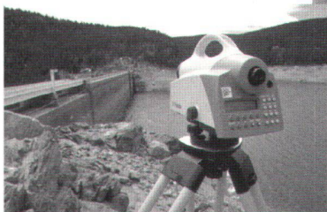
Trimble DiNi12 - Digitalnivellier
