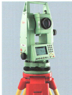
Fig. 1: Série TPS700 Performance. Tachéomètres légers et compacts pour mesurer avec rapidité, efficacité et confort.
