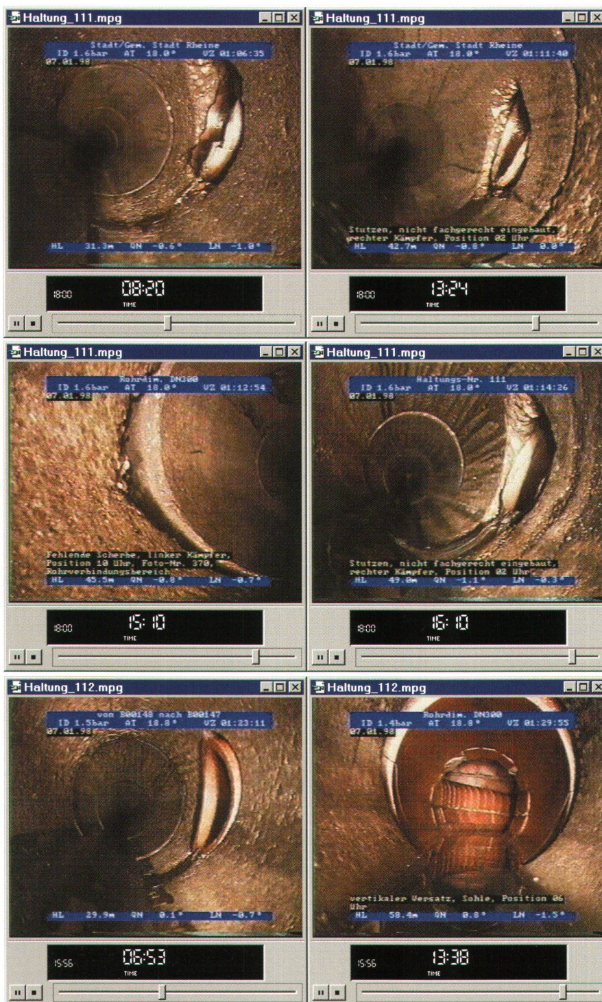
Abb. 3: Kanalisationen.
