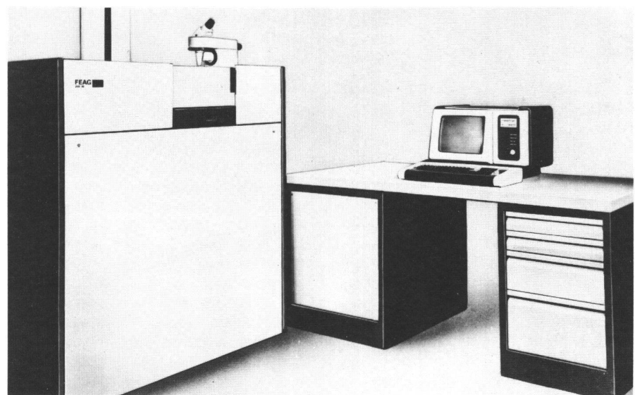
Abb. 1 Filmein-/Ausgabe-Gerät FEAG links: Grundgerät mit mechanisch-optischer Lasereinheit, Elektroniksteuerung mit Mikrorechnersystem rechts: Bedienterminal und Koppereinheit mit Controllern
