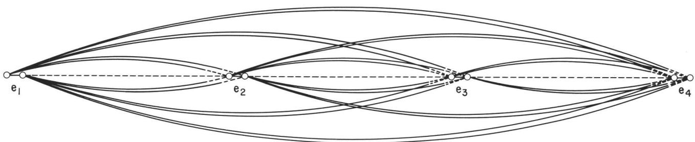
Abb. 4 Bestimmung der Additionskorrektur eines EDM-Gerätes mit Hilfe von drei unbekannten Teilstrecken
