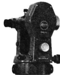
Kern DKM 2-A Sekundentheodolit mit automatischer Höhenkollimation
