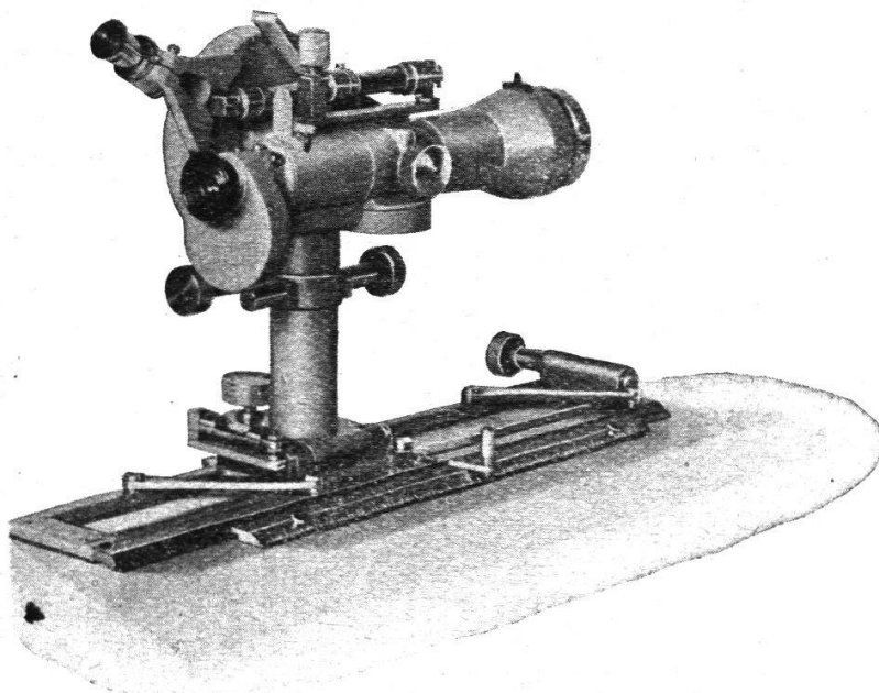
Kippregel Nr. 79
