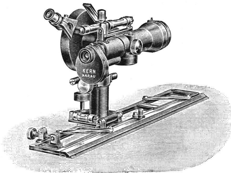
Kippregel Nr. 79
