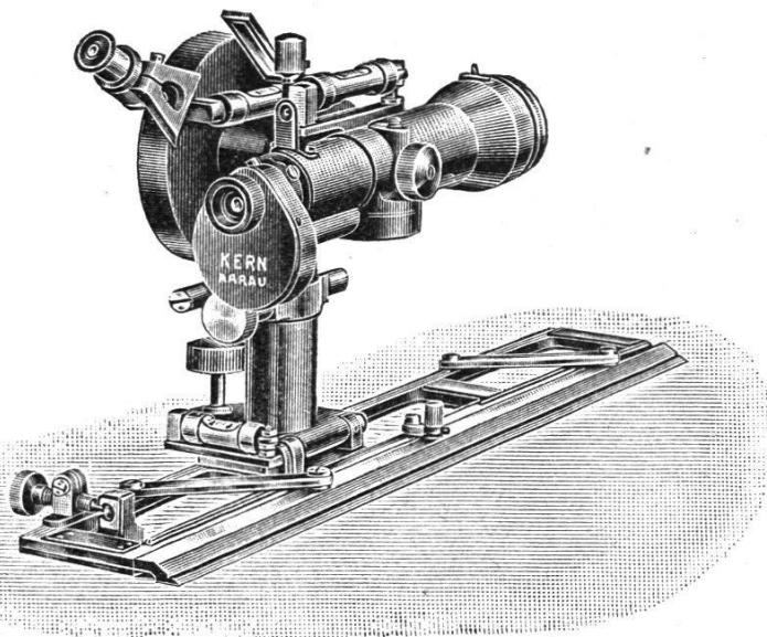
Kippregel Nr. 79
