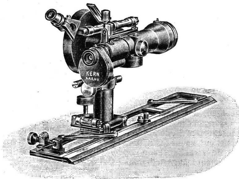
Kippregel Nr. 79
