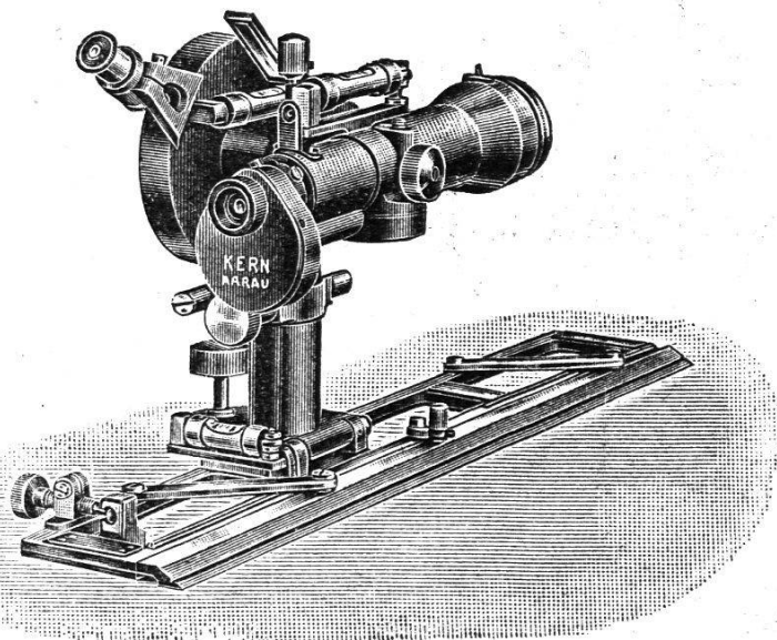
Kippregel Nr. 79
