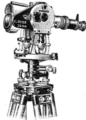
Reduktions-Tachymeter
