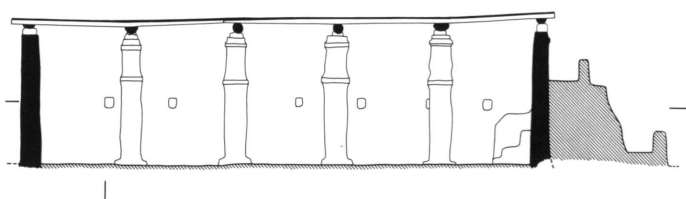
Coupe A-A
