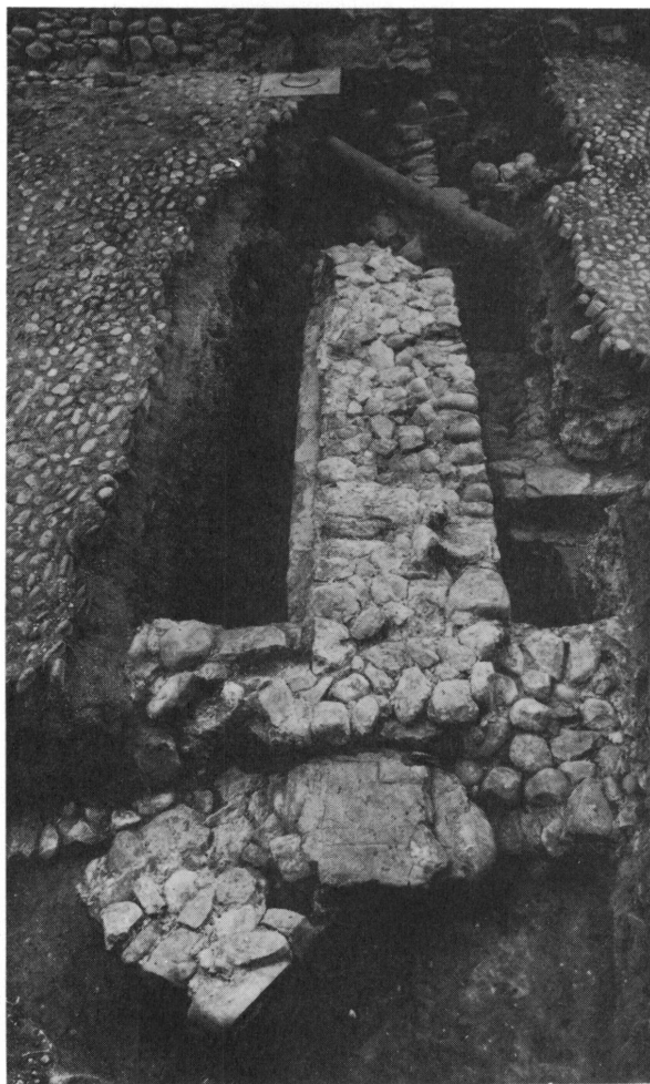
Figure 30. Mur mitoyen de la première et de la deuxième chapelle.
