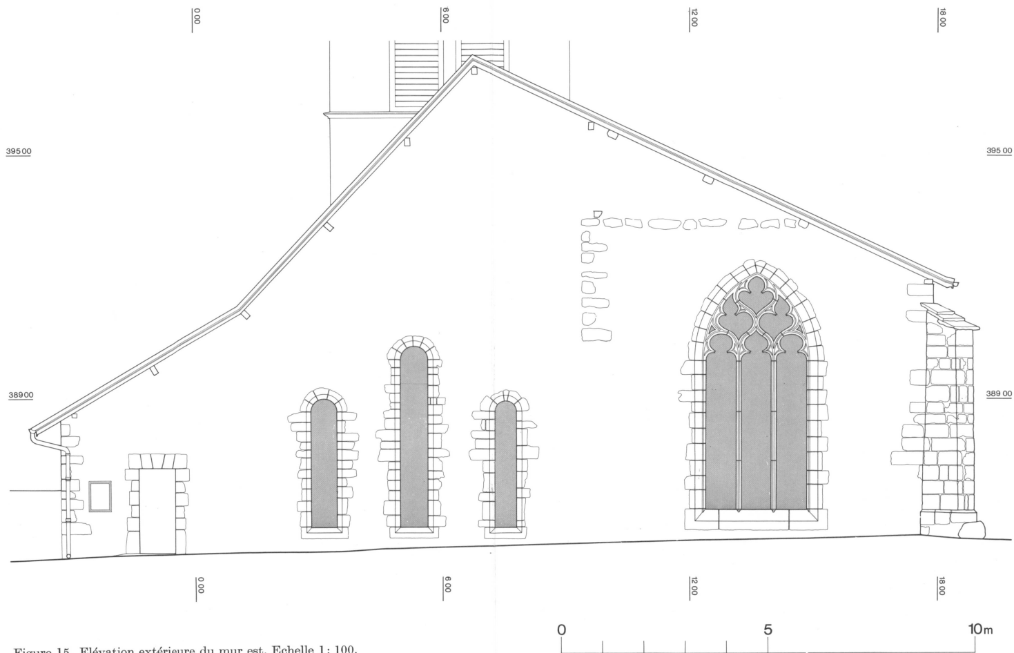
Figure 15. Elévation extérieure du mur est. Echelle 1: 100.
