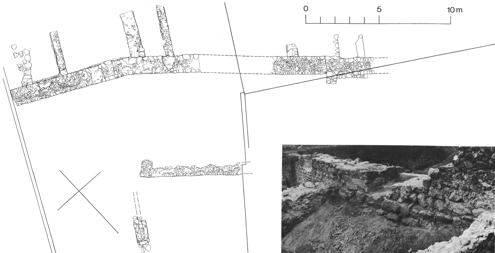
Figure 8. Rempart nord du Bourg-d'en-Bas, plan des fouilles de 1972. Vue de la poterne.
