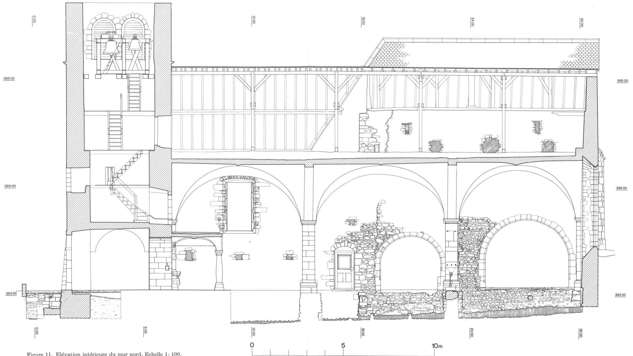
Figure 11. Elévation intérieure du mur nord. Echelle 1: 100.
