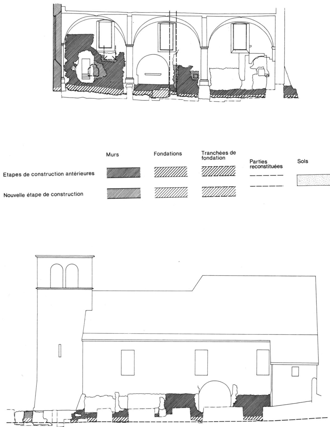
Figure 37. Eglise du xv e siècle. Schéma des élévations du mur sud. Echelle 1: 250.
