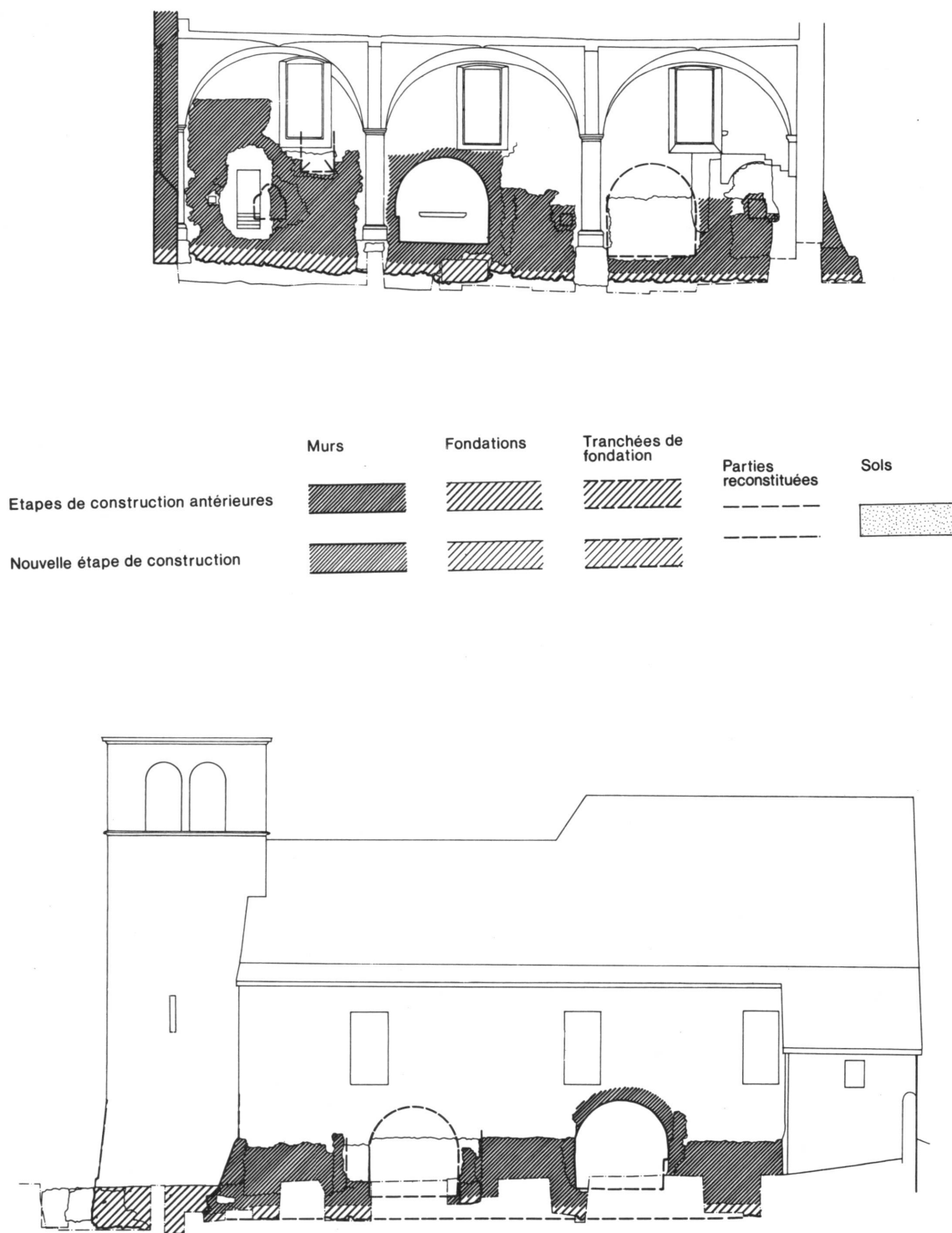
Figure 40. Eglise du x v e siècle et chapelle de la Visitation. Schéma des élévations du mur sud. Echelle 1 : 250.
