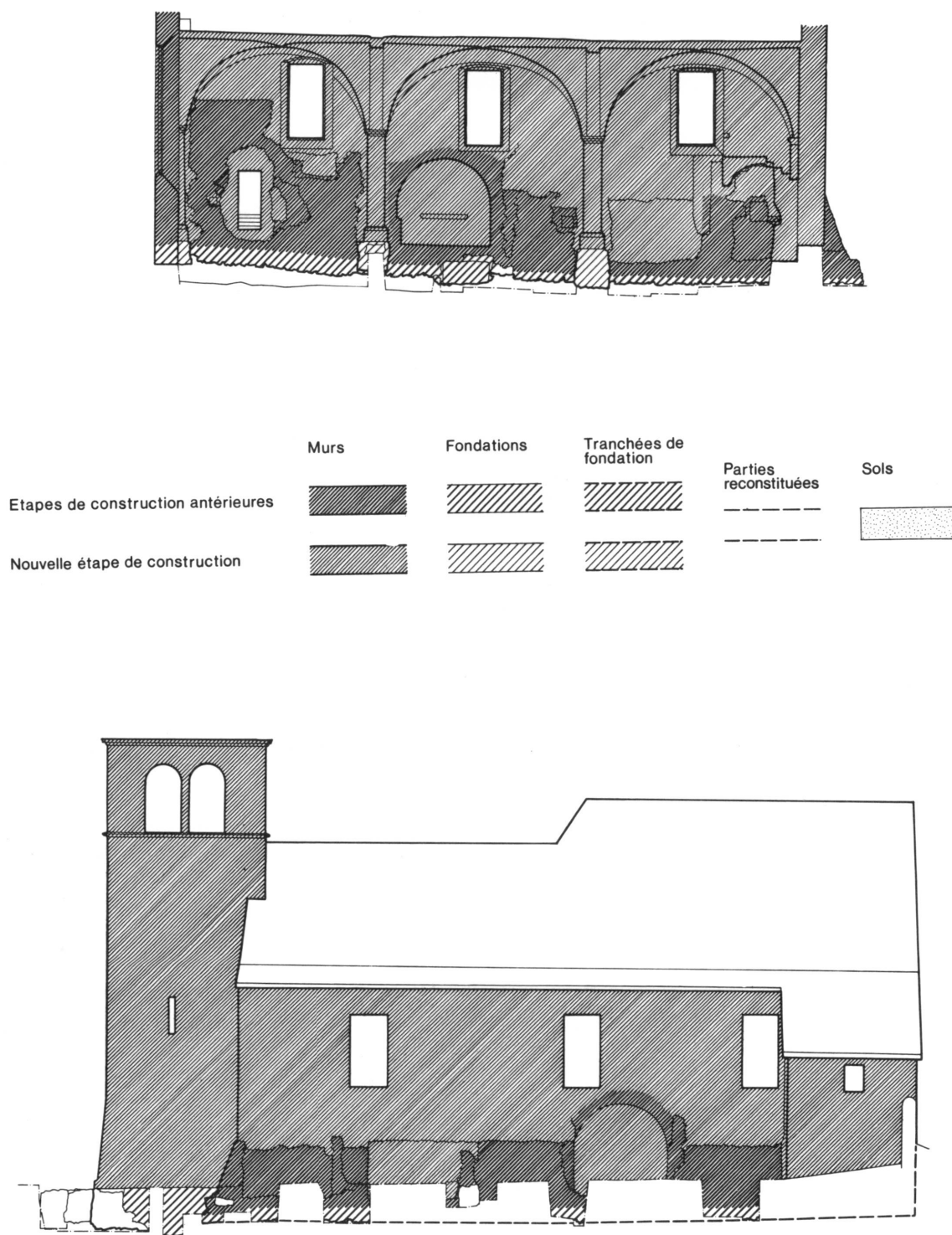
Figure 43. Eglise de 1679. Schéma des élévations du mur sud. Echelle 1 : 250.
