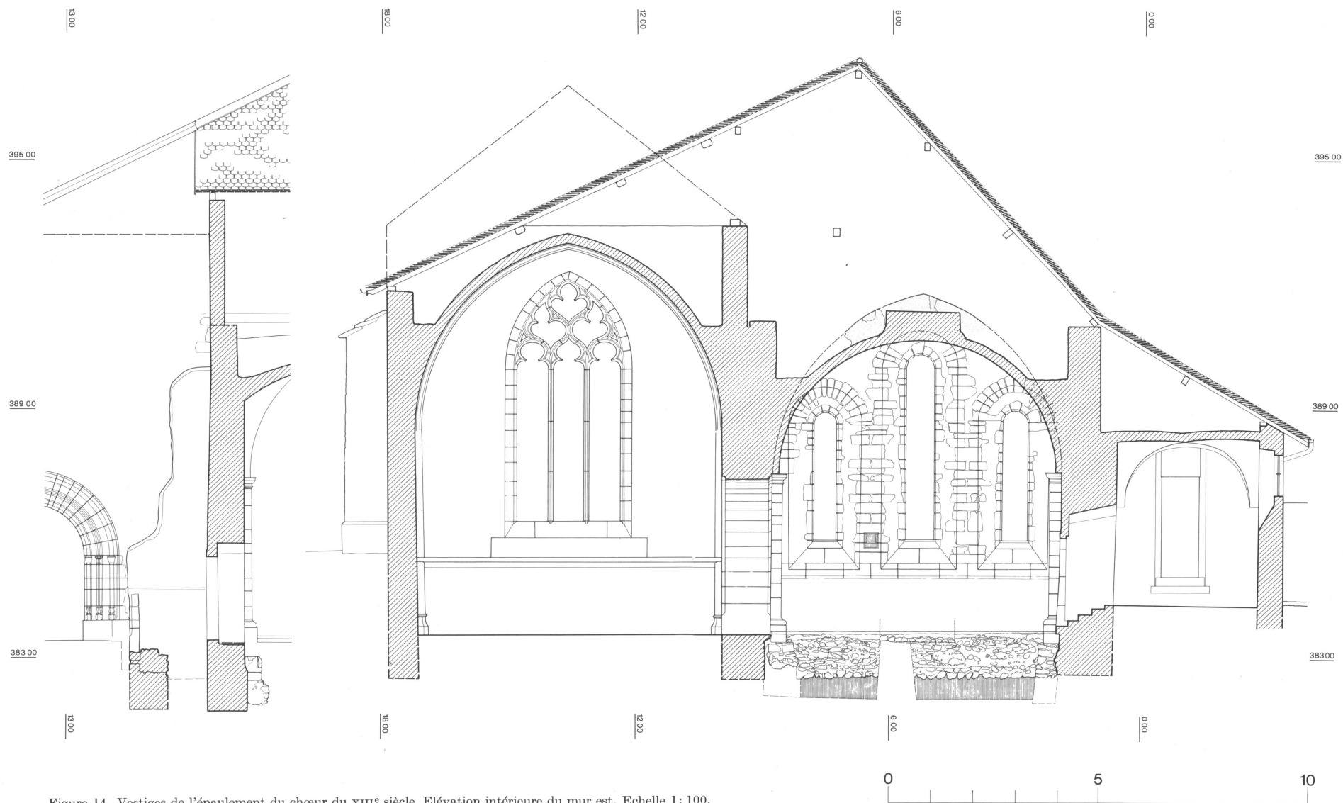
Figure 14. Vestiges de l'épaulement du chœur du XIII e siècle. Elévation intérieure du mur est. Echelle 1: 100.
