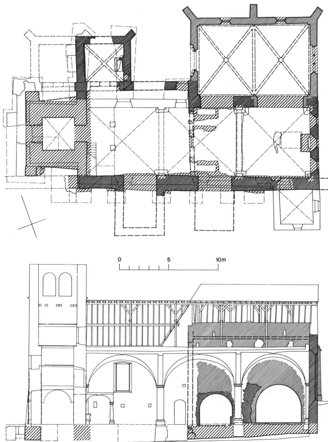
Figure 39. Eglise du x v e siècle et chapelle de la Visitation. Schéma du plan et de l'élévation intérieure nord. Echelle 1: 250.
