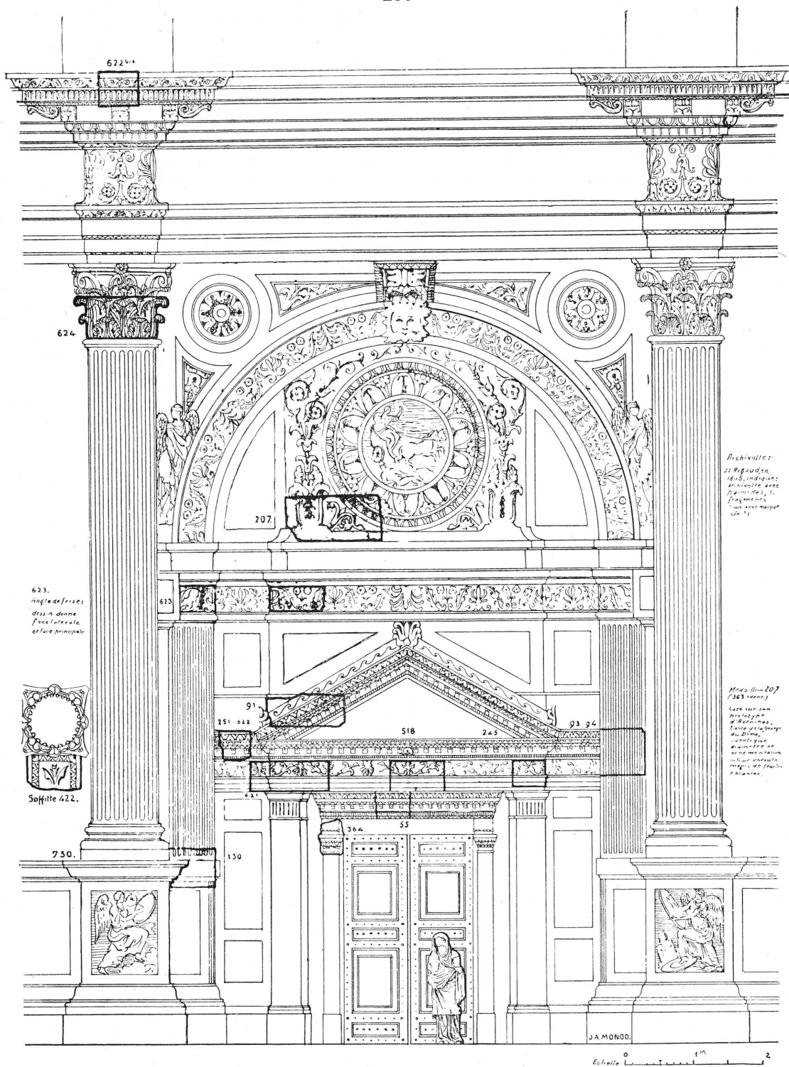
Reconstitution d'une porte monumentale, à laquelle pourraient convenir les fragments suivants : pilastres 158 (130), 159 (93-4); fronton 171 (91); architrave et soffit 174 (422); frise et architrave 178 (518); angle de frise 179 (623); frise 180 (621); grand pilastre d'ordre corinthien 181 (624); frise et architrave 185 (245); petit chapiteau de pilastre 195 (364); corniche 203 (251); 204 (55); médaillon et décor floral 207 (207); corniche 208 (622); 209 (622bis), 216 (730).
