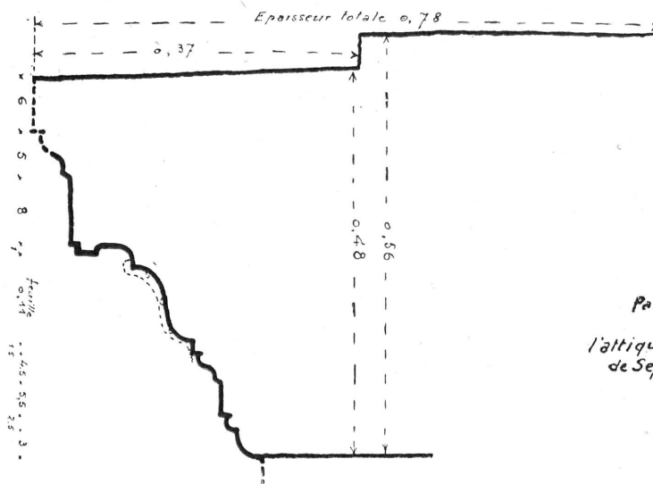
N° 175. — Fragment de corniche, profil.
