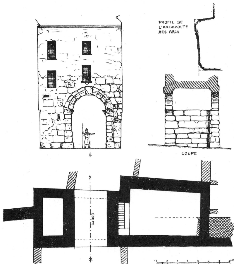
Porte romaine du Bourg-de-Four, d'après M. L. Blondel.
