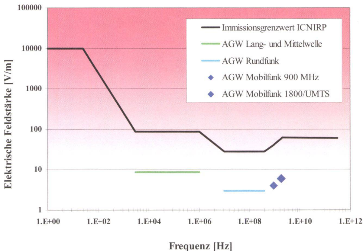
Figur 1: Grenzwerte für das elektrische Feld in Abhängigkeit der Frequenz des EMF nach 20 .
