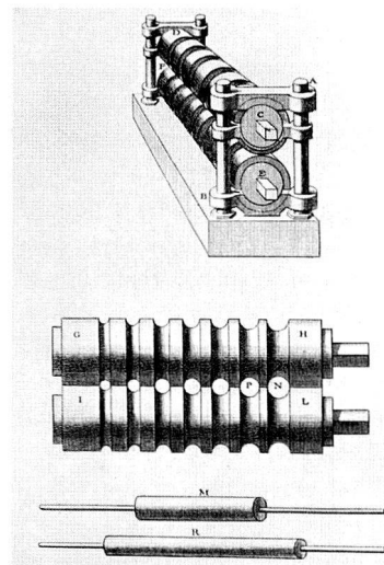
Bild 13: Umkehrwalzwerk für Blei- und Kupferbleche mit Rollgang; Drehrichtungswechsel mittels Umschaltkupplung; um 1730.
