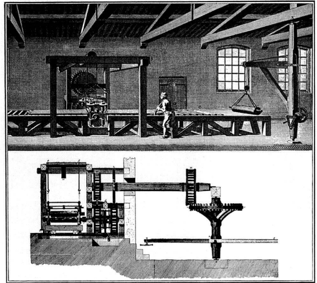
Bild 13: Umkehrwalzwerk für Blei- und Kupferbleche mit Rollgang; Drehrichtungswechsel mittels Umschaltkupplung; um 1730.
