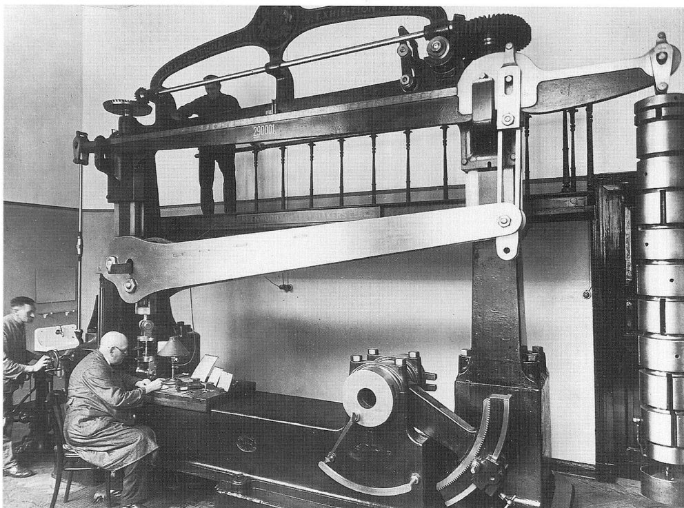
Zerreißmaschine für die mechanische Werkstoffprüfung. Alfred Krupp hat diese Universalprüfmaschine 1862 auf der Londoner Weltausstellung erworben.
