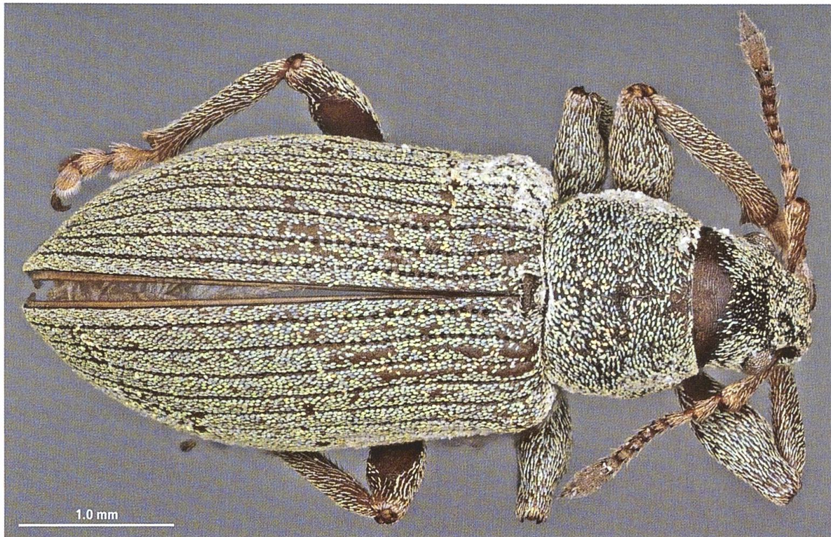
Abb. 1. Habitus von Polydrusus abeillei abeillei , Männchen Trient, coll. N. Cerutti. (Foto Christoph Germann)
