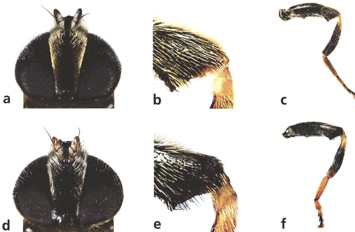
Fig. 2. Merodon gallicus Vujić & Radenković, 2012, femelle : a) tête, b) appendice triangulaire du fémur postérieur, c) patte postérieure. Merodon ruficornis Meigen, 1822, femelle : d) tête, e) appendice triangulaire du fémur postérieur, f) patte postérieure. (Photos M.C.D. Speight)
