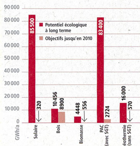
Graphique 1: potentiels à long terme écologiquement acceptables des énergies renouvelables suisses: électricité
