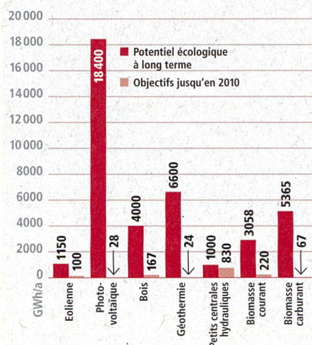
Graphique 2: potentiels à long terme écologiquement acceptables des énergies renouvelables suisses: chaleur
