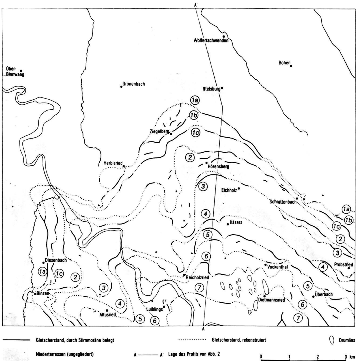
Fig. 1. Die Gletscherstände des würmzeitlichen Iller-Gletschers auf Blatt 8127 Grönenbach 1:25.000 und die Lage des Blattes im deutschen Alpenvorland. Aus Habbe 1985 (Reproduktion mit Bewilligung von Quartär).
