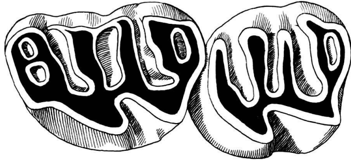
Fig. 2. Blainvillimys gregarius SCHLOSSER 1884. BHM: 1879 XV 605: D 4 -M 1 (Escamps). × 14,5.
