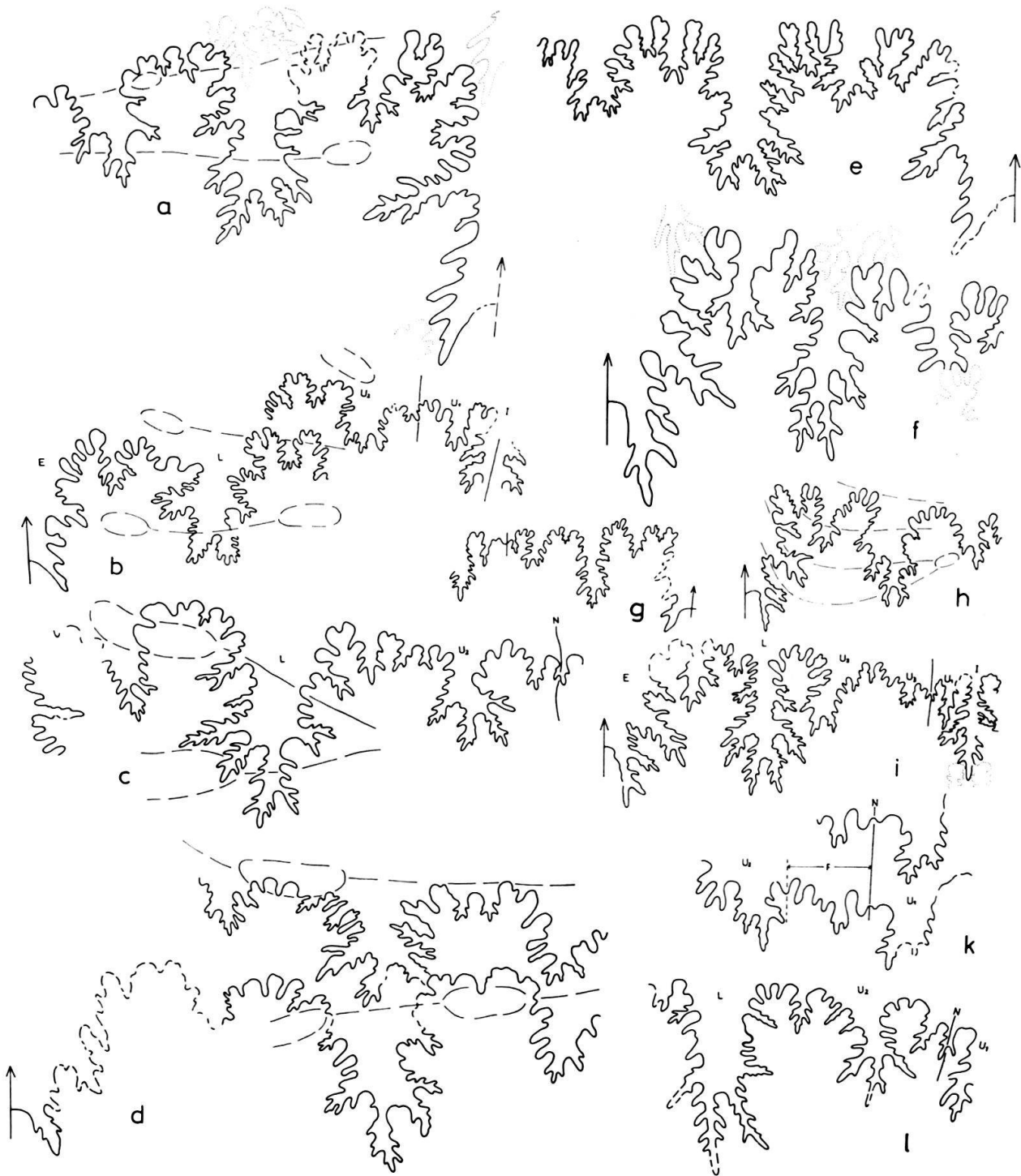
Fig. 7. Suturlinien von Mortonicerias . Wo nichts bemerkt, nat. Gr.
