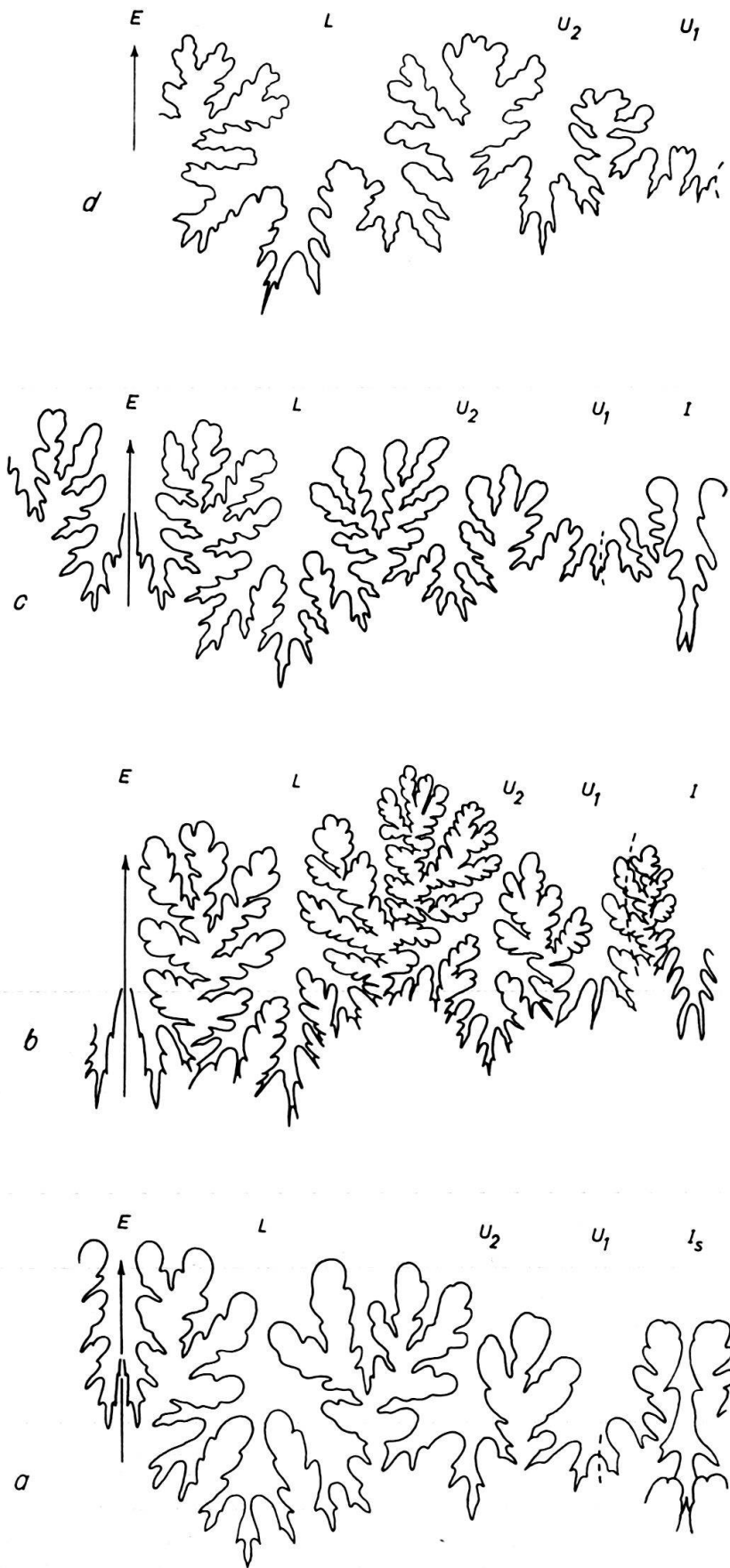
Fig. 9. Die Lytoceraten-Nebenlinien. a: Gesamtsutur von Pleuroacanthites biformis (J. SOWERBY) [n. CANAVARI 1888, Textfig. 2], Hettangien, Spezia (Italien). b: Gesamtsutur von Ectocentrites petersi (HAUER), Holotyp [n. WÄHNER 1898, Taf. 62, Fig. 5], Hettangien, Kammerkaralpe (Österr.). c: Gesamtsutur von Eolytoceras tasekoi FREBOLD, Paratypoid GSC 20060, Unteres Hettangien, Taseko-Seengebiet (Kanada). Bei Wh 18 mm. d: Externsutur von Peltolytoceras giordanii (BONARELLI), Hypotyp. IGT (leg. BONARELLI), Sinemurien, Ponte Alto (Foci di Cagli, Zentralapennin). Bei Wh 18 mm.
