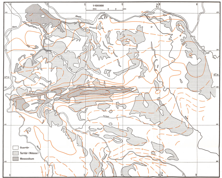
«BOUGUERKARTE II» Kurven gleicher Werte von u_i in mg/l.
