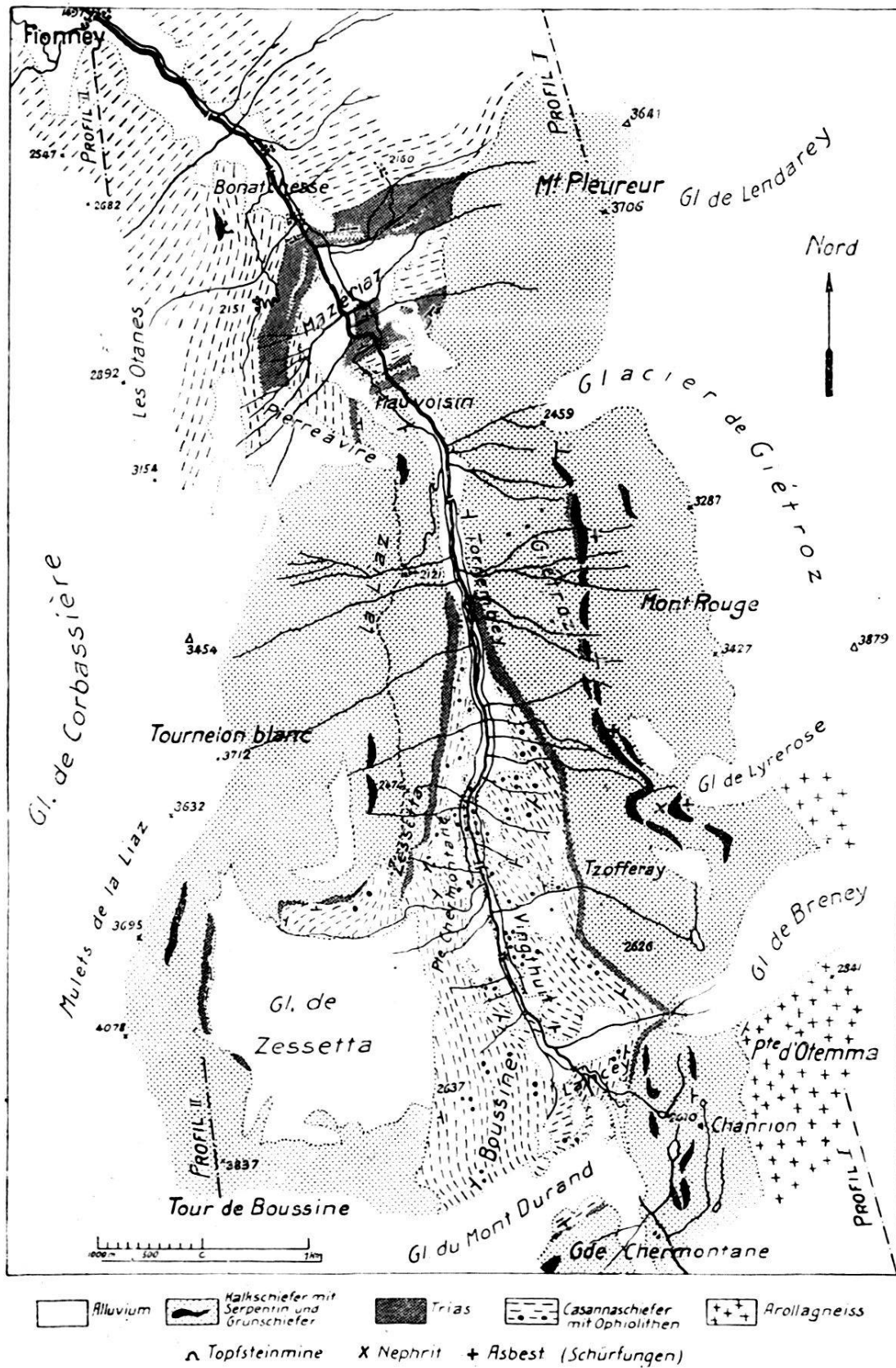
Geologische Karte des Oberen Val de Bagnes.
