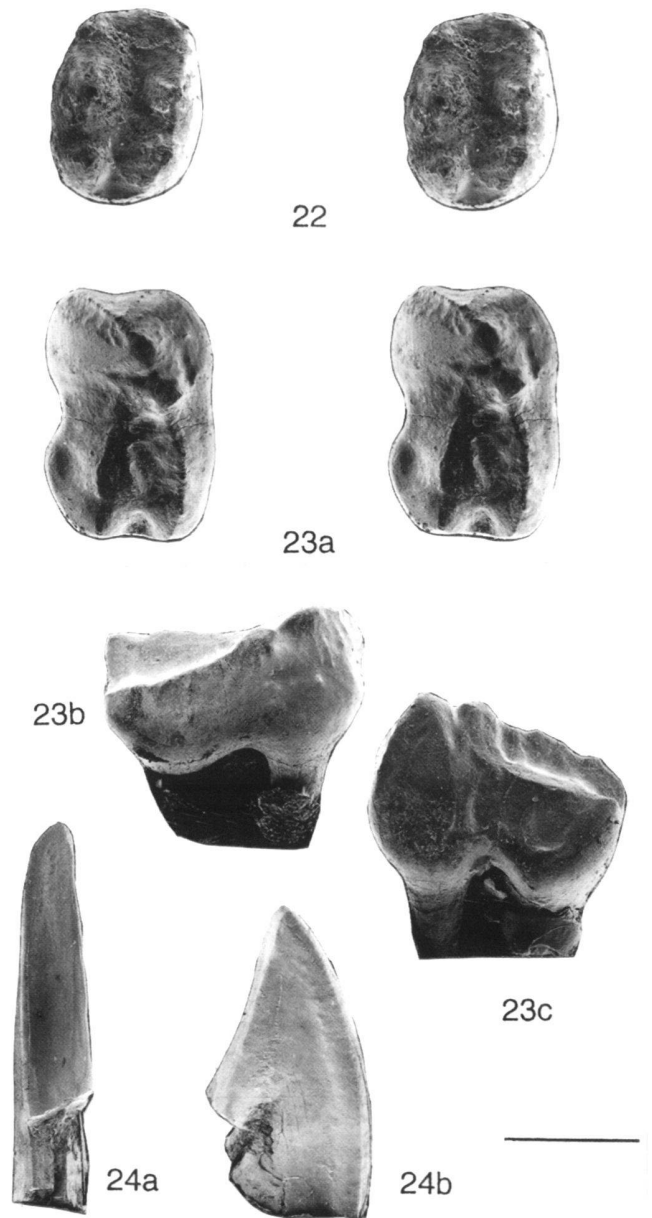
Fig. 22–23. cf. Hainina sp. Fig. 22: JBA-4, P3/ en vue occlusale (stéréo); fig. 23a–c: dP4/? en vues occlusale (stéréo), linguale et labiale. Echelle = 1 mm.
