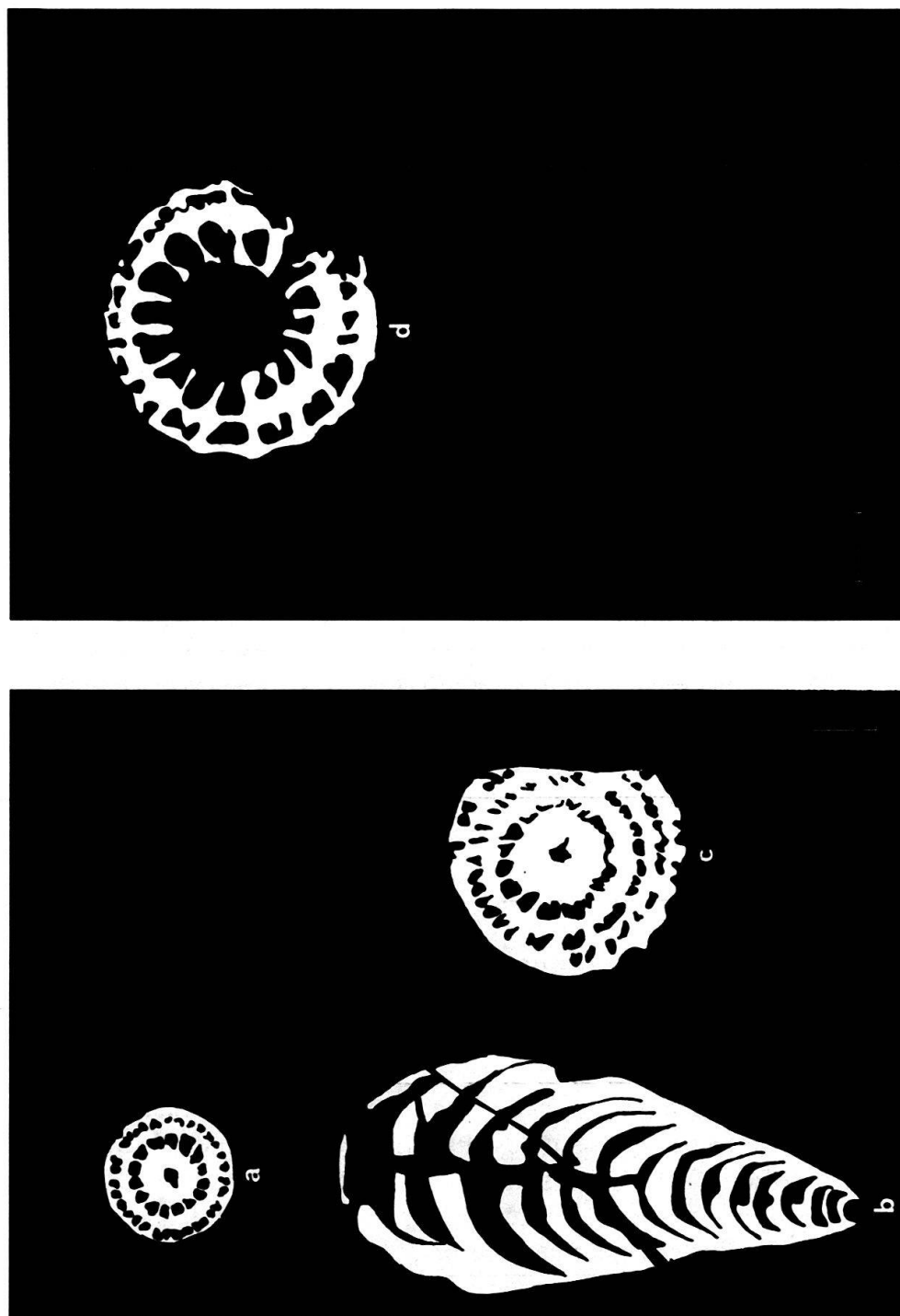
Fig. 1. Coupe d'Episcopi (Hydra, Grèce): Colaniella ex gr. lepada WANG.
